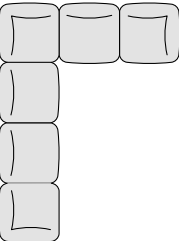
31KC1 W: 2400 D: 800 H: 430 Angular section D: 3200
