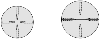
41E01 Ø: 1200 H: 730/900/1060 41E02 Ø: 1400 H: 730/900/1060
