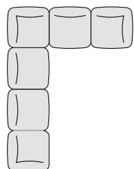
31KC1 W: 2400 D: 800 H: 378 Angular section D: 3200
